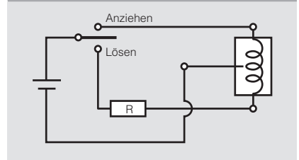
Schaltbild 2
