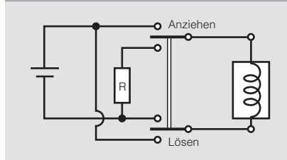
Schaltbild 1
